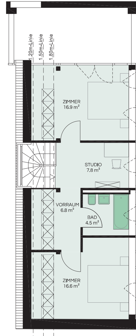
1. OBERGESCHOSS
