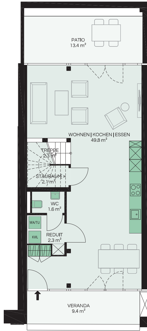
ERDGESCHOSS
