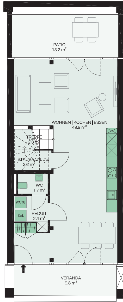
ERDGESCHOSS
