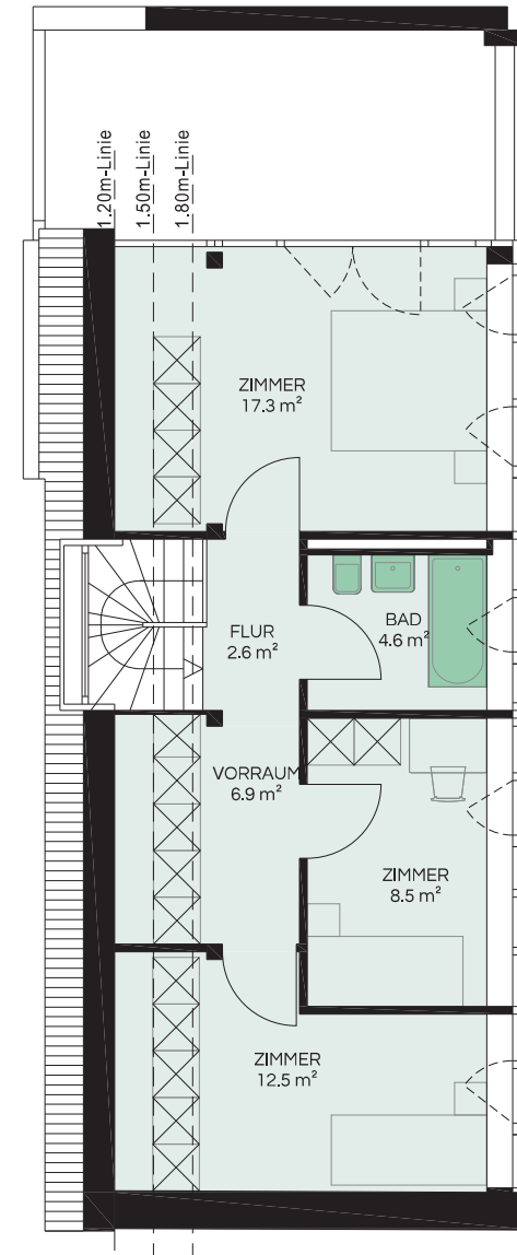
1. OBERGESCHOSS
