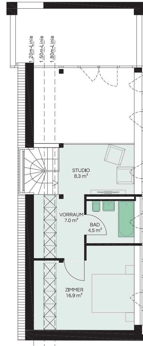
1. OBERGESCHOSS
