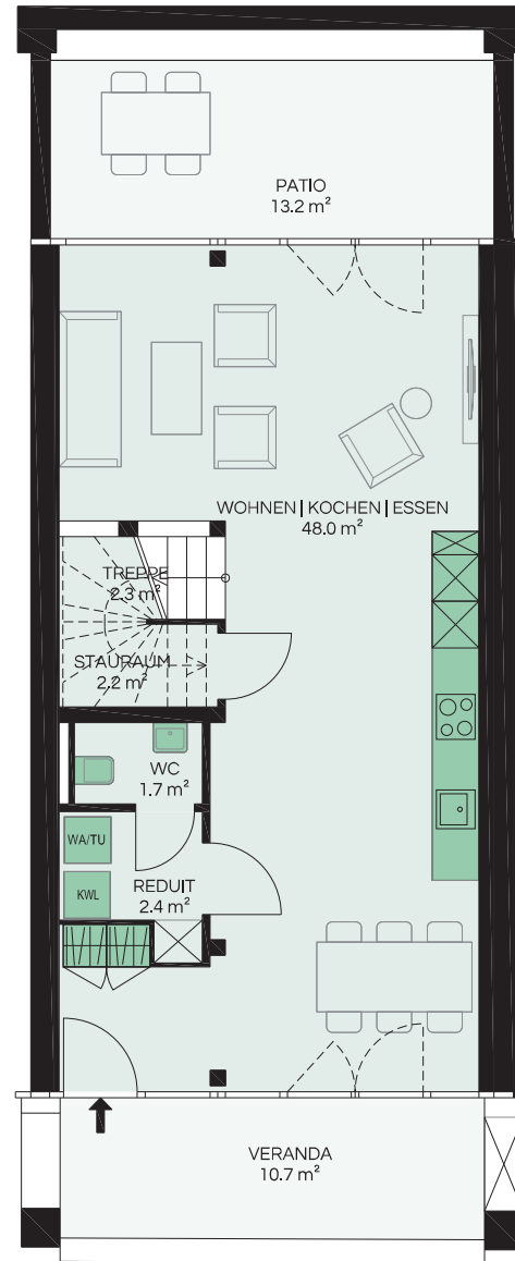
ERDGESCHOSS
