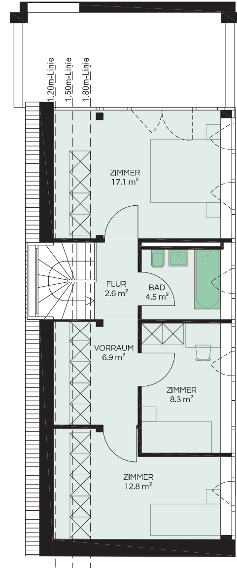
1. OBERGESCHOSS
