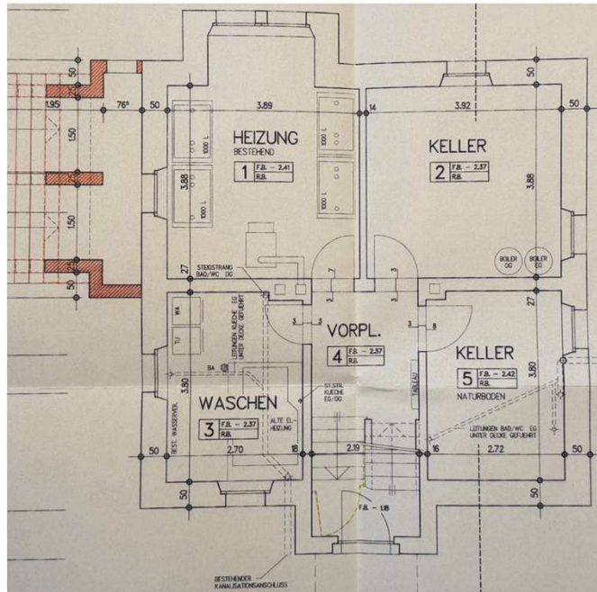
Untergeschoss
