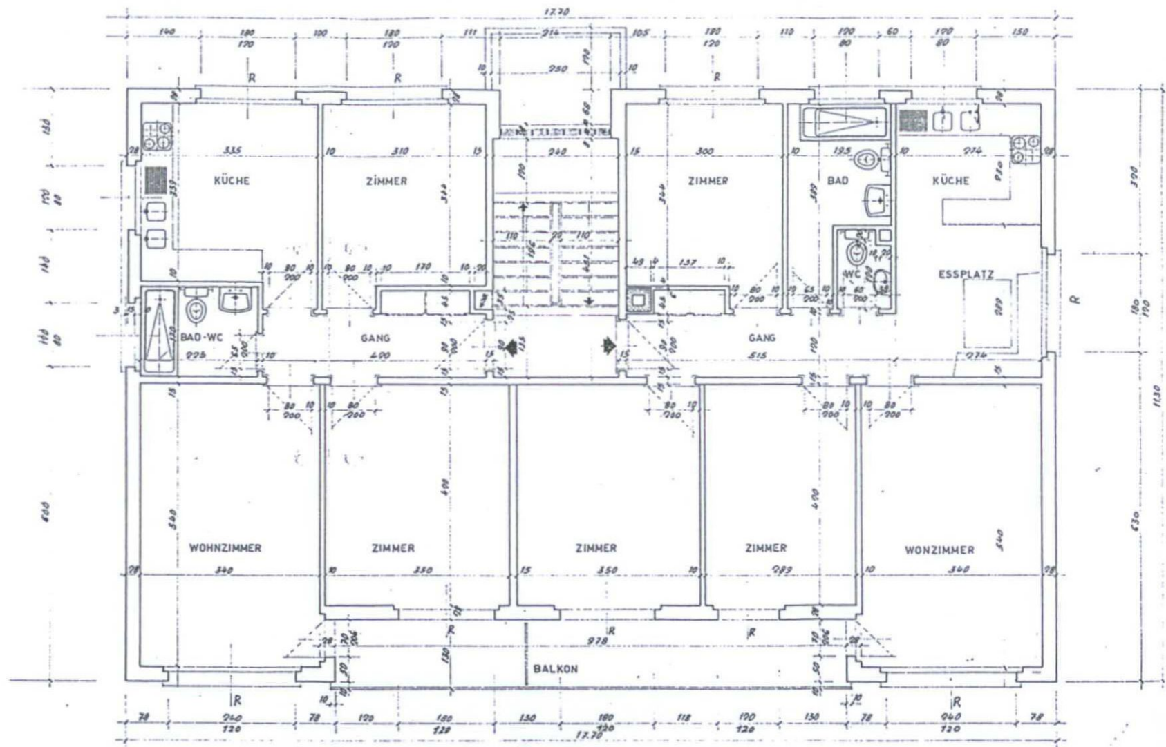
2. OBERGESCHOSS
