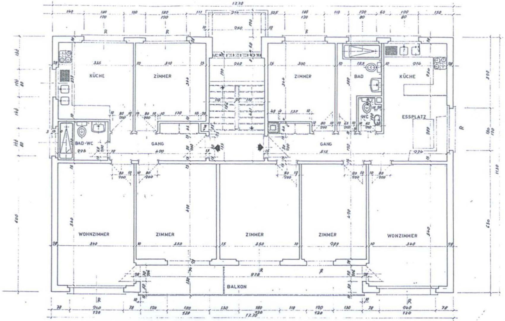
1. OBERGESCHOSS
