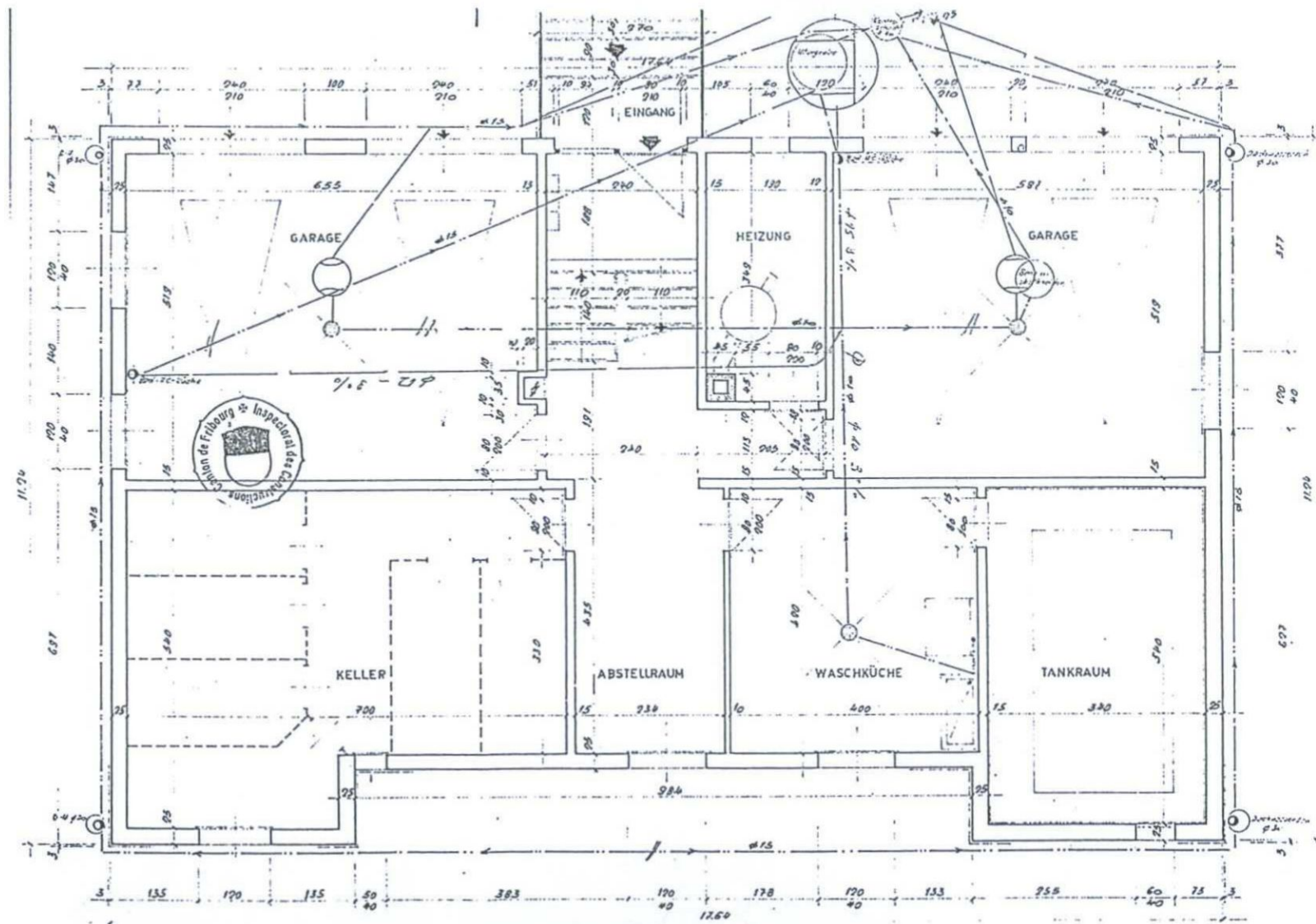
KELLERGESCHOSS
