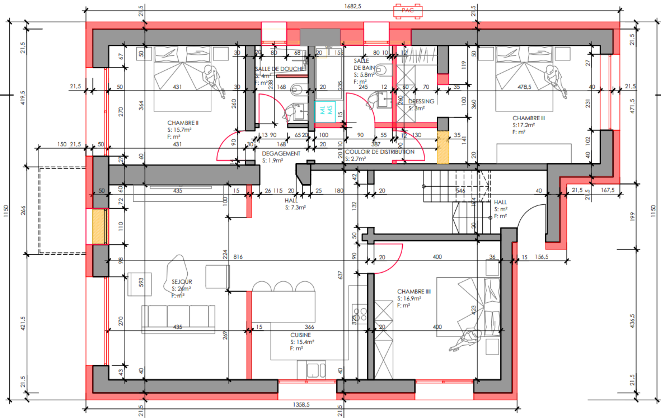
PLAN REZ-DE-CHAUSSEE 1:100
