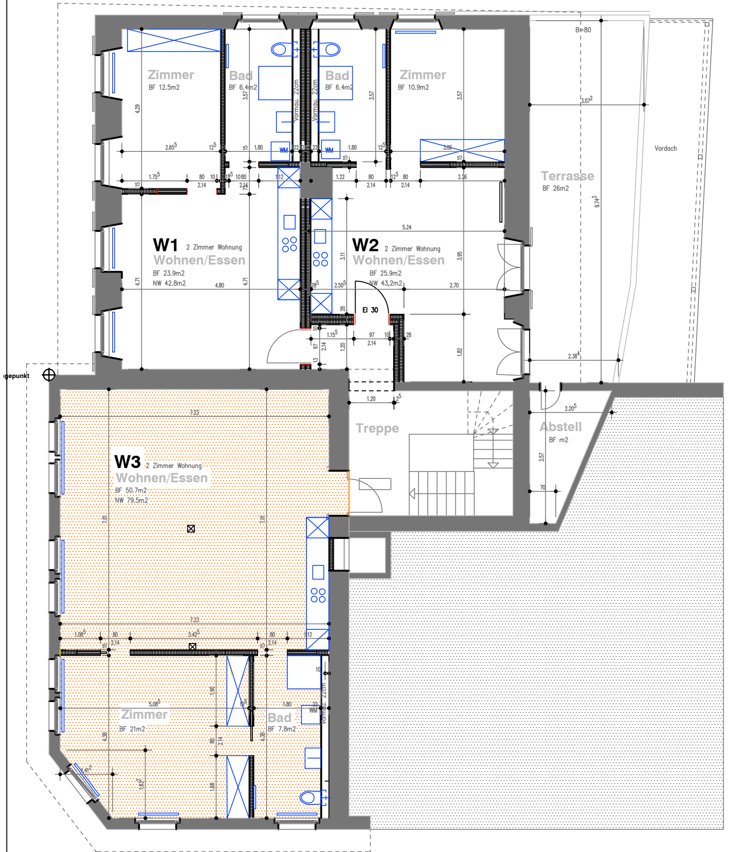
Mietwohnungen Rössli Wohnung 3 Obergeschoss 1:100
