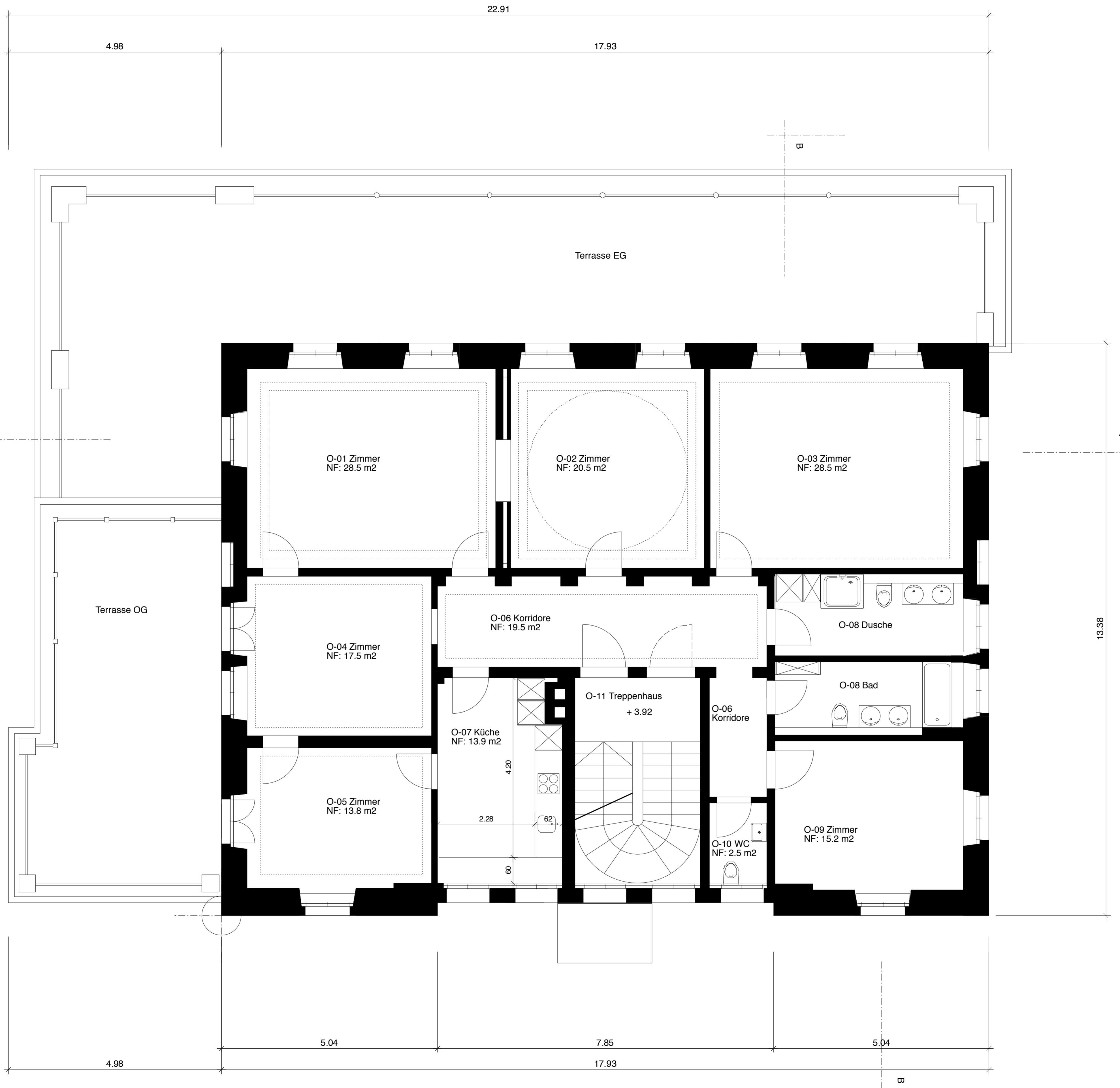
1. Obergeschoss
