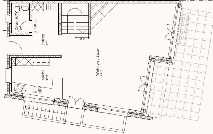
Erdgeschoss
