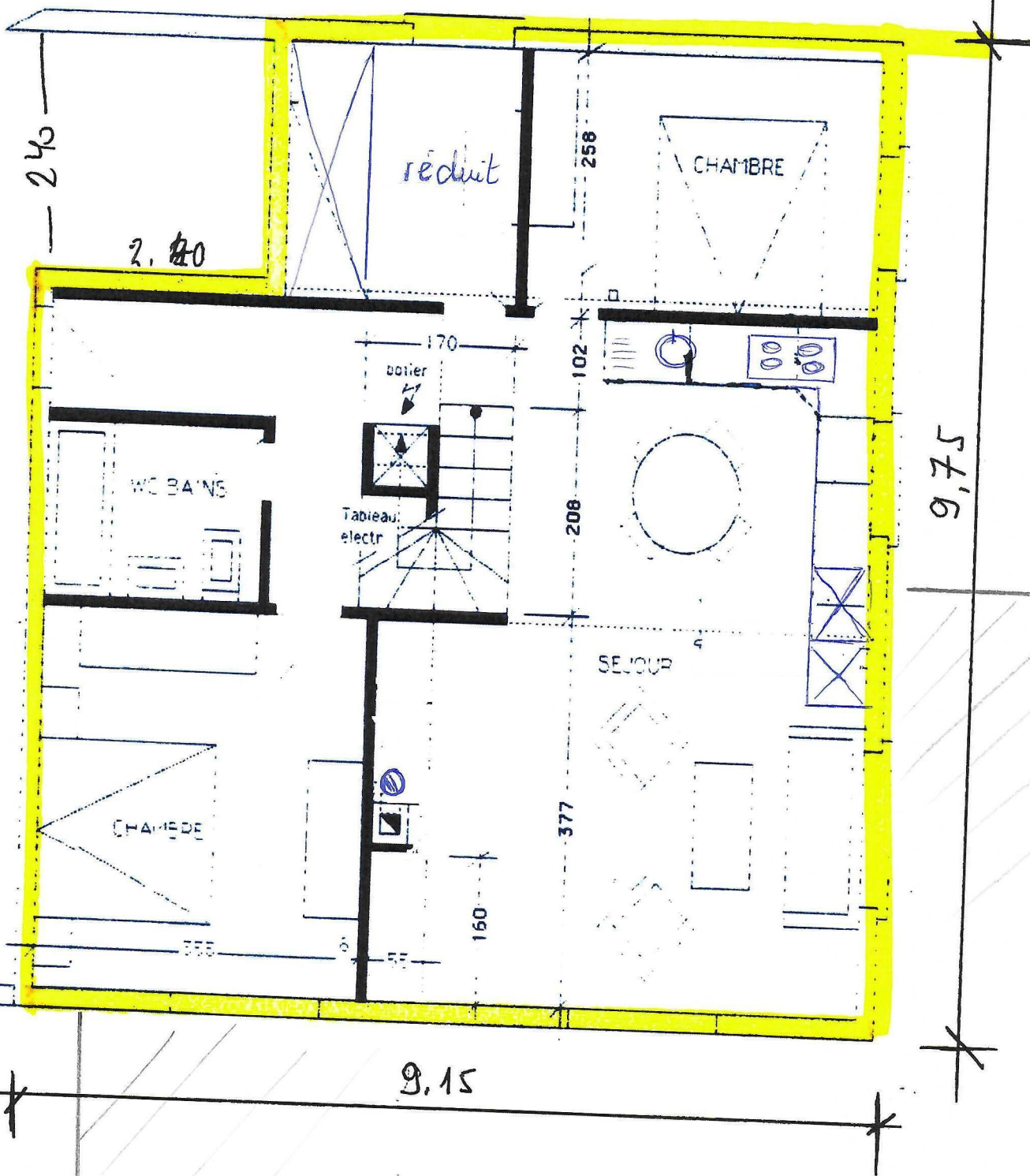
Plan de l'étage - éch. 1:50
