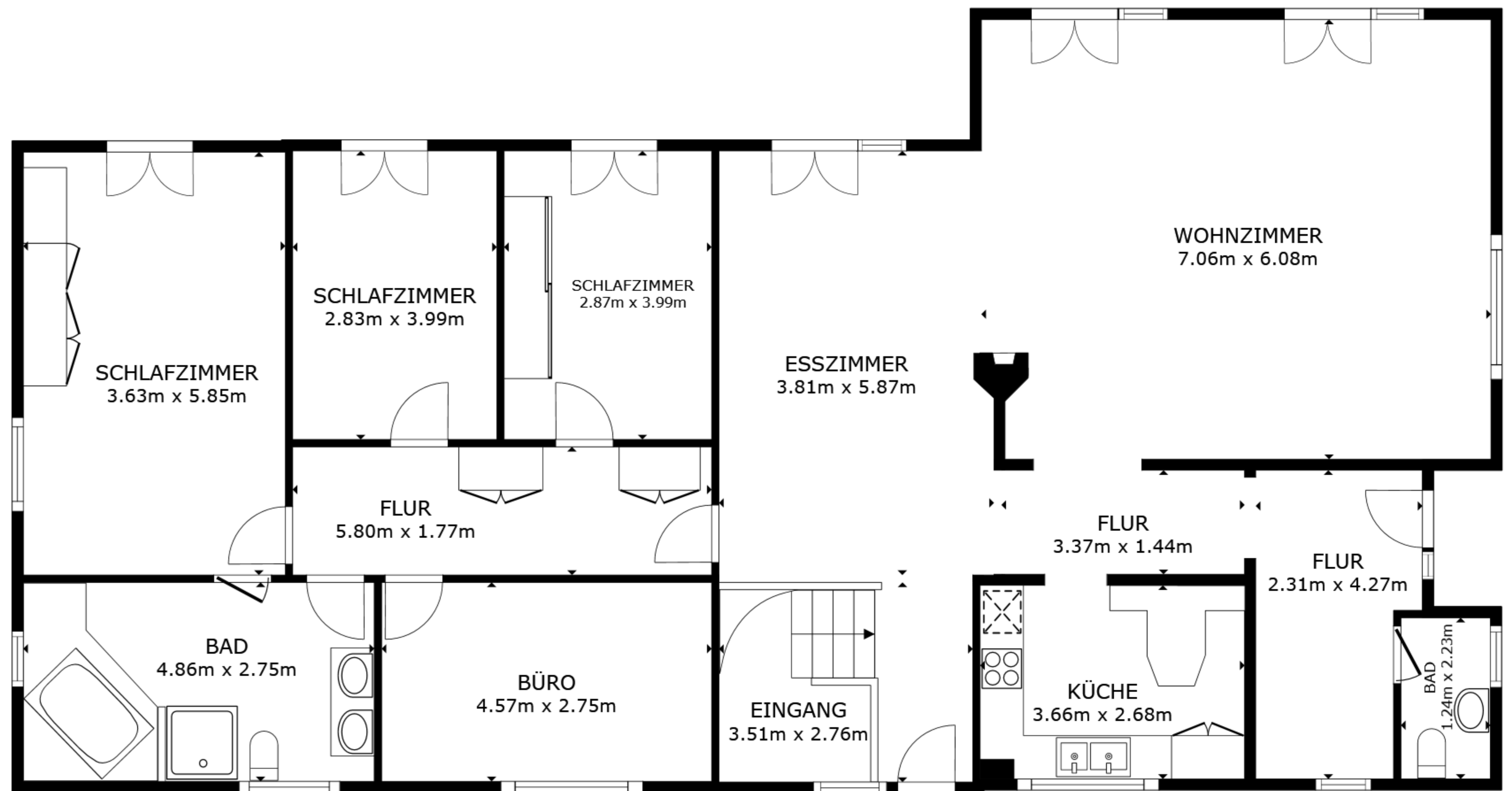
STOCKWERK 2
